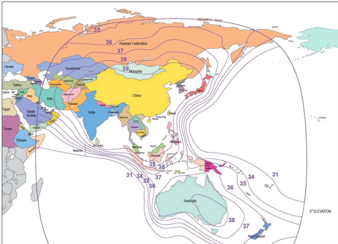
亞洲四號衛星(東經 122 度) C 波段 EIRP (dBW)
