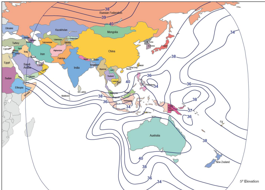
亞洲六號衛星(東經 120 度)C 波段 EIRP (dBW)
